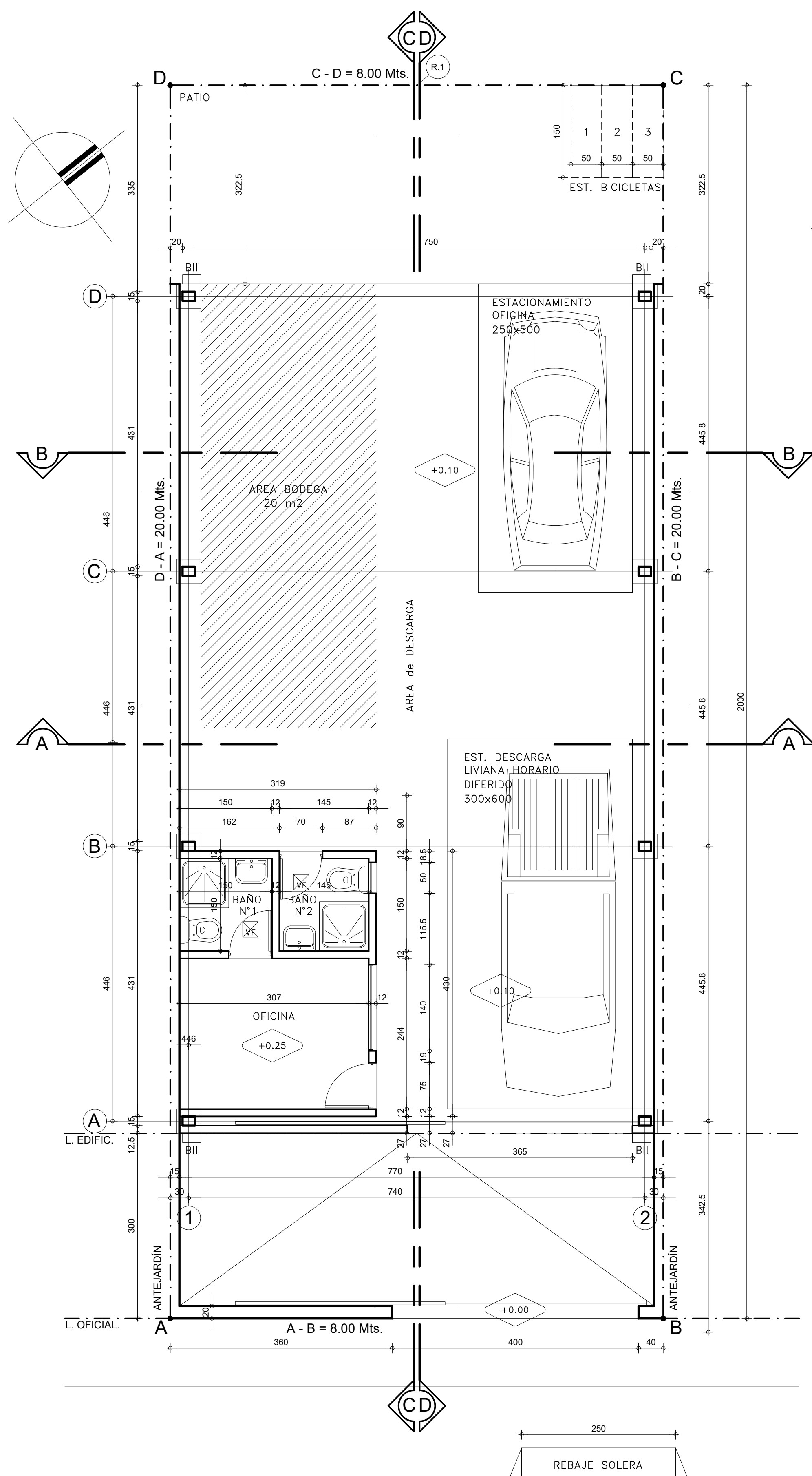
1 PLANTA ARQUITECTURA 1:50
